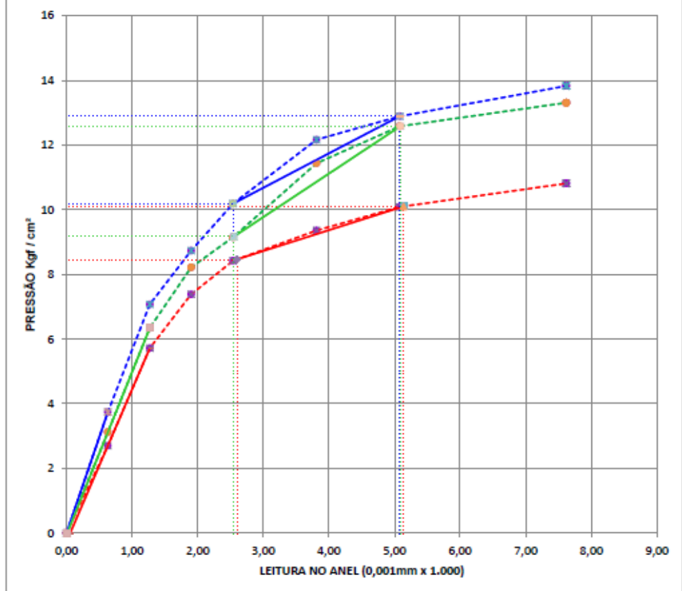
GRÁFICO DE PRESSÃO E PENETRAÇÃO
