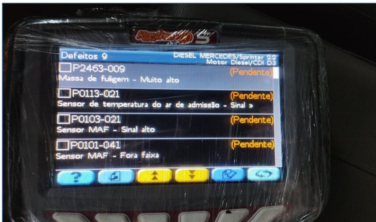
IMAGEM DE SCANNER EXECUTADO NO VEÍCULO
