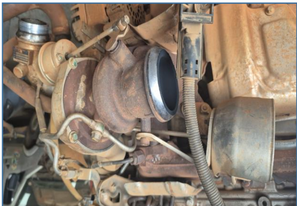
IMAGEM DA TURBINA DA VAN, A MESMA FOI TESTADA
