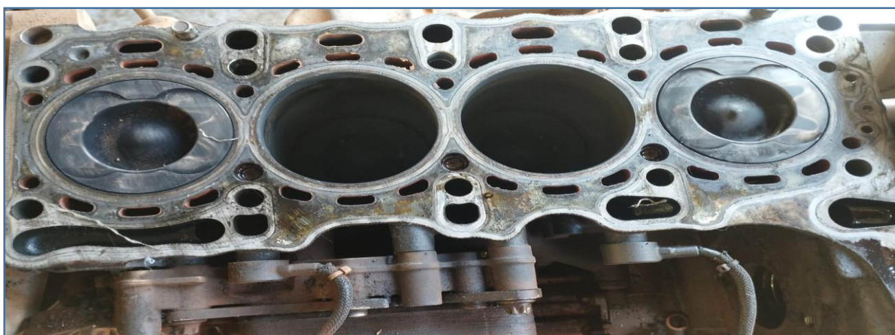
IMAGEM LADO "B" DO CABEÇOTE DO VEÍCULO QUE FOI DESMONTADO PARA VERIFICAÇÃO
