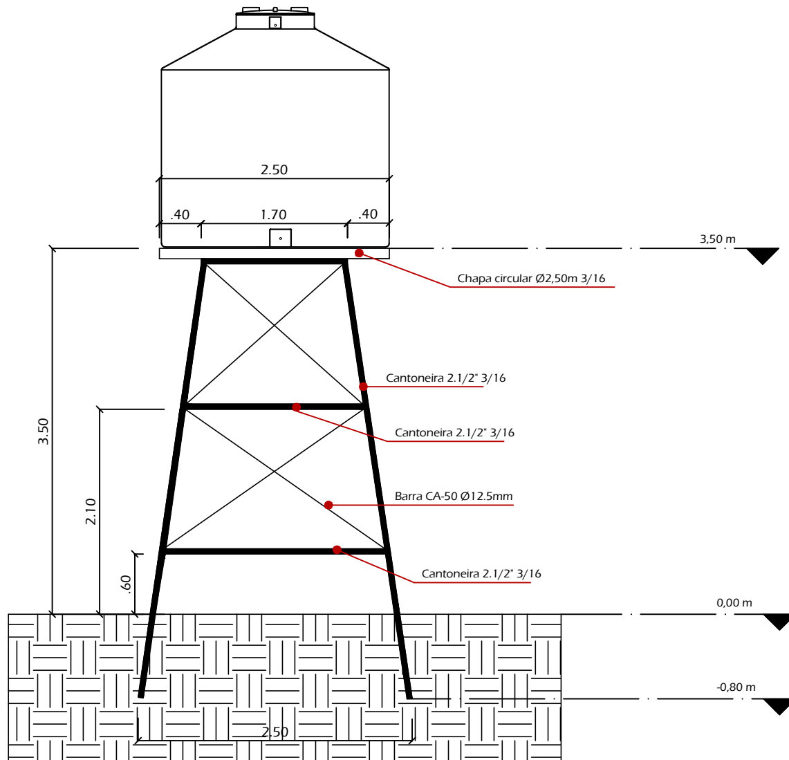
01 Vista Frontal Escala 1/50
