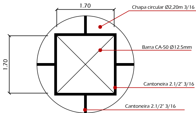
01 Planta Baixa Escala 1/50
